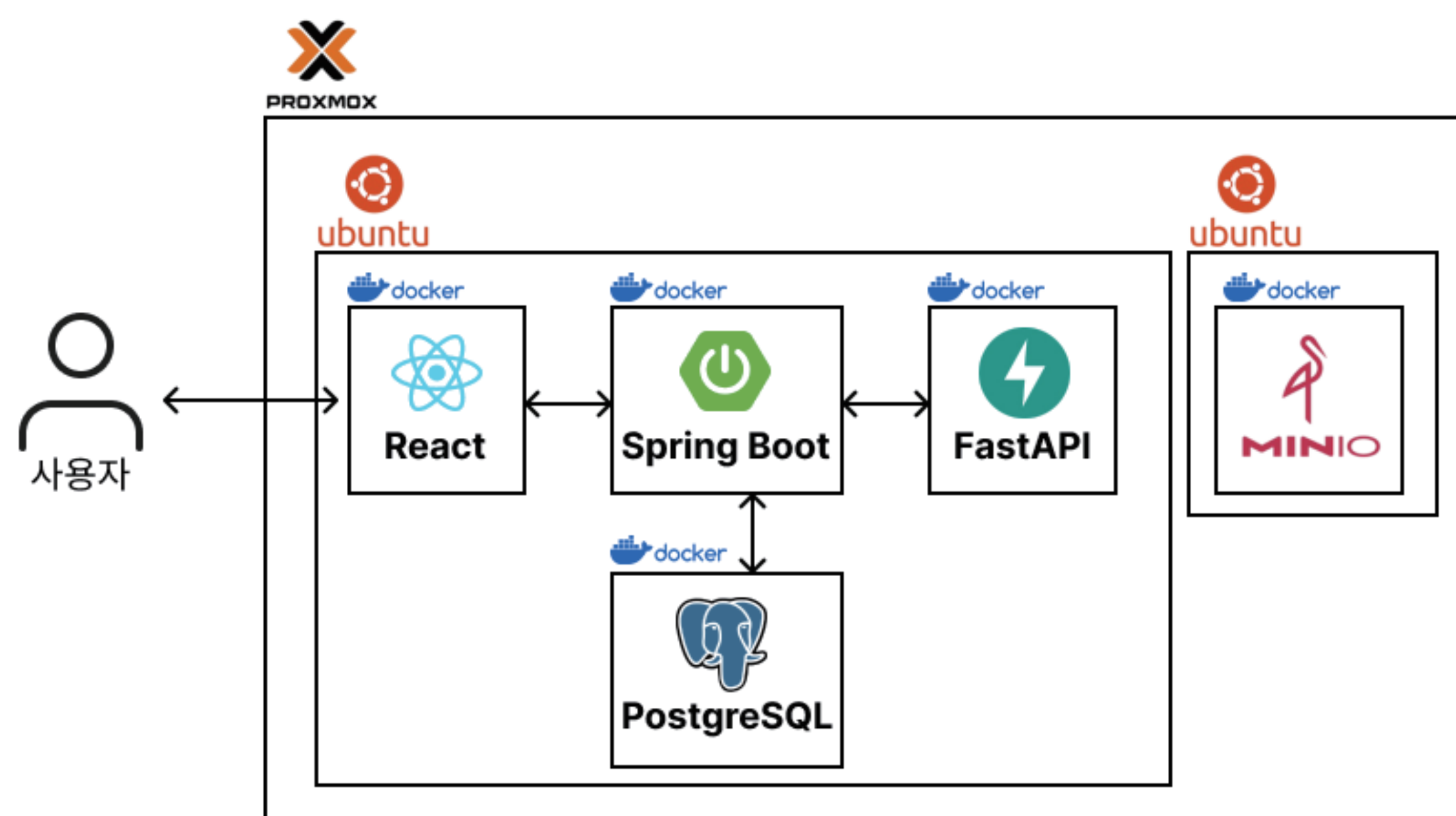
개발구성도
