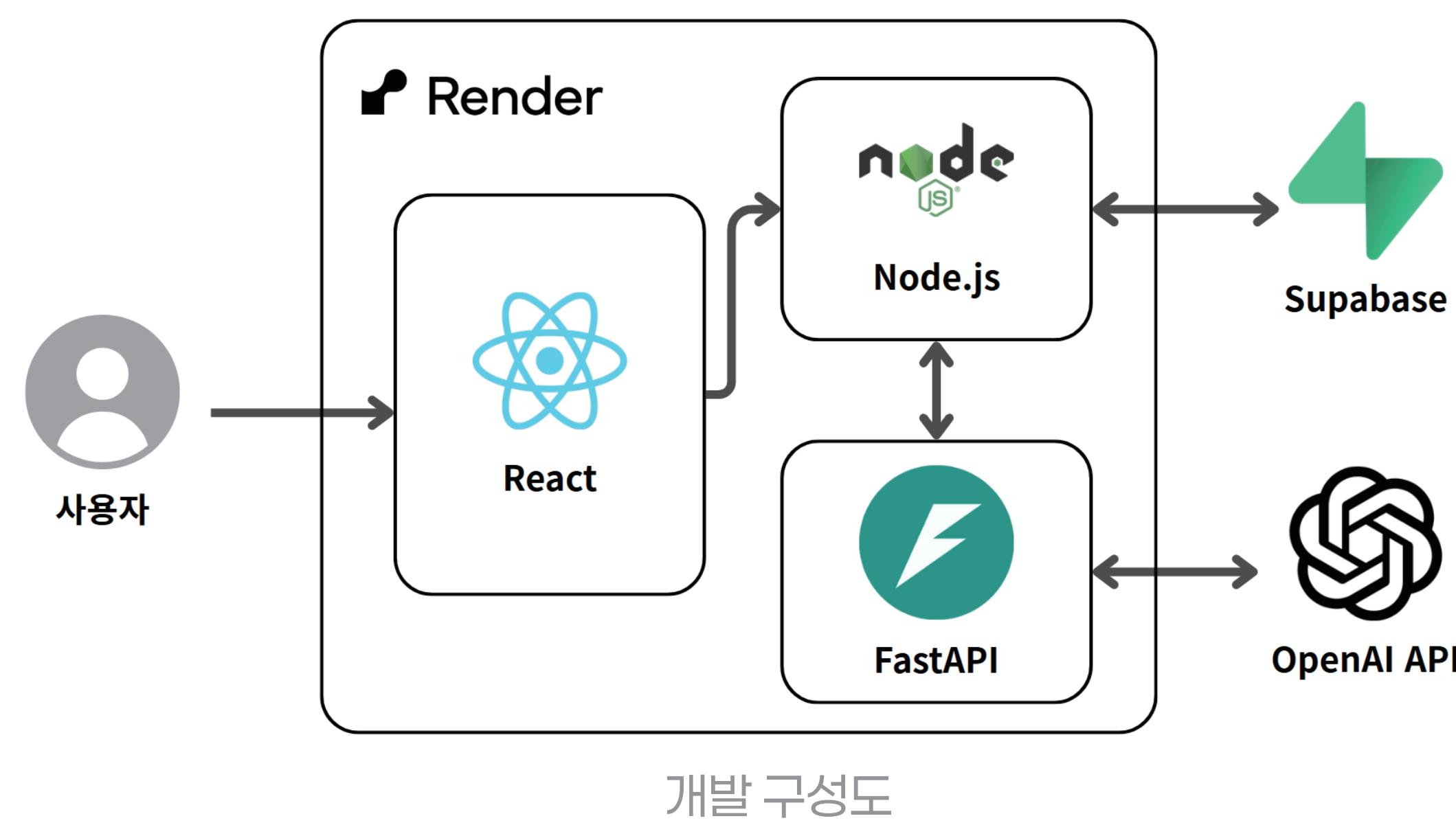
개발 구성도
