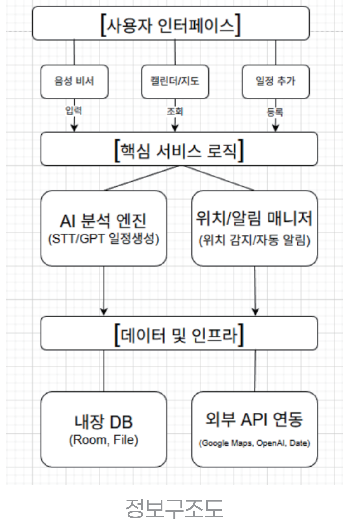
정보구조도
