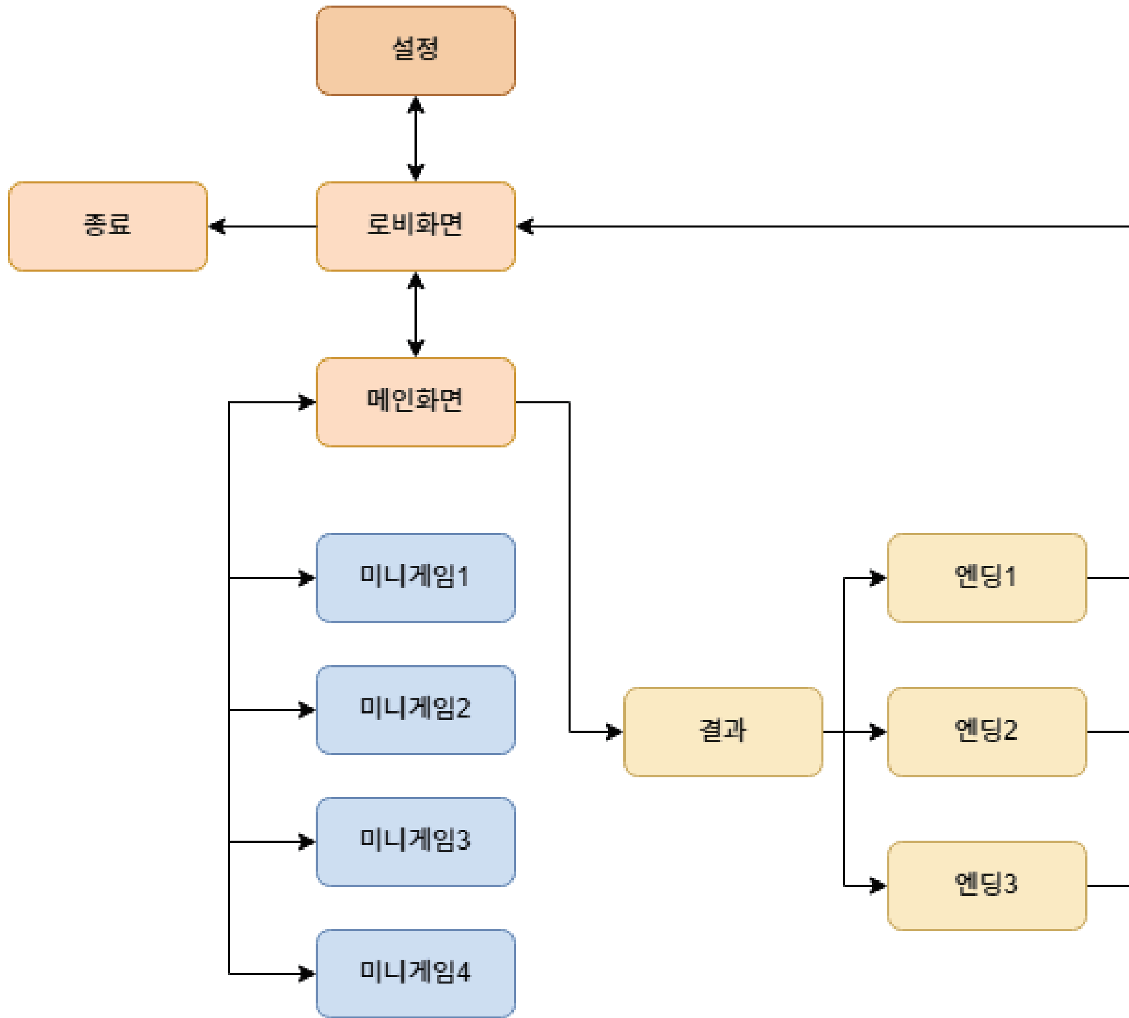
정보구조도
