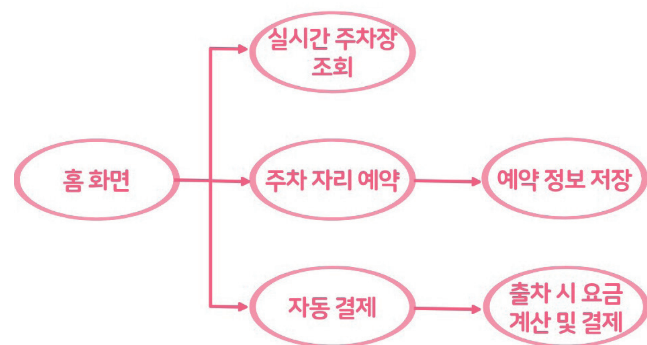
정보구조도
