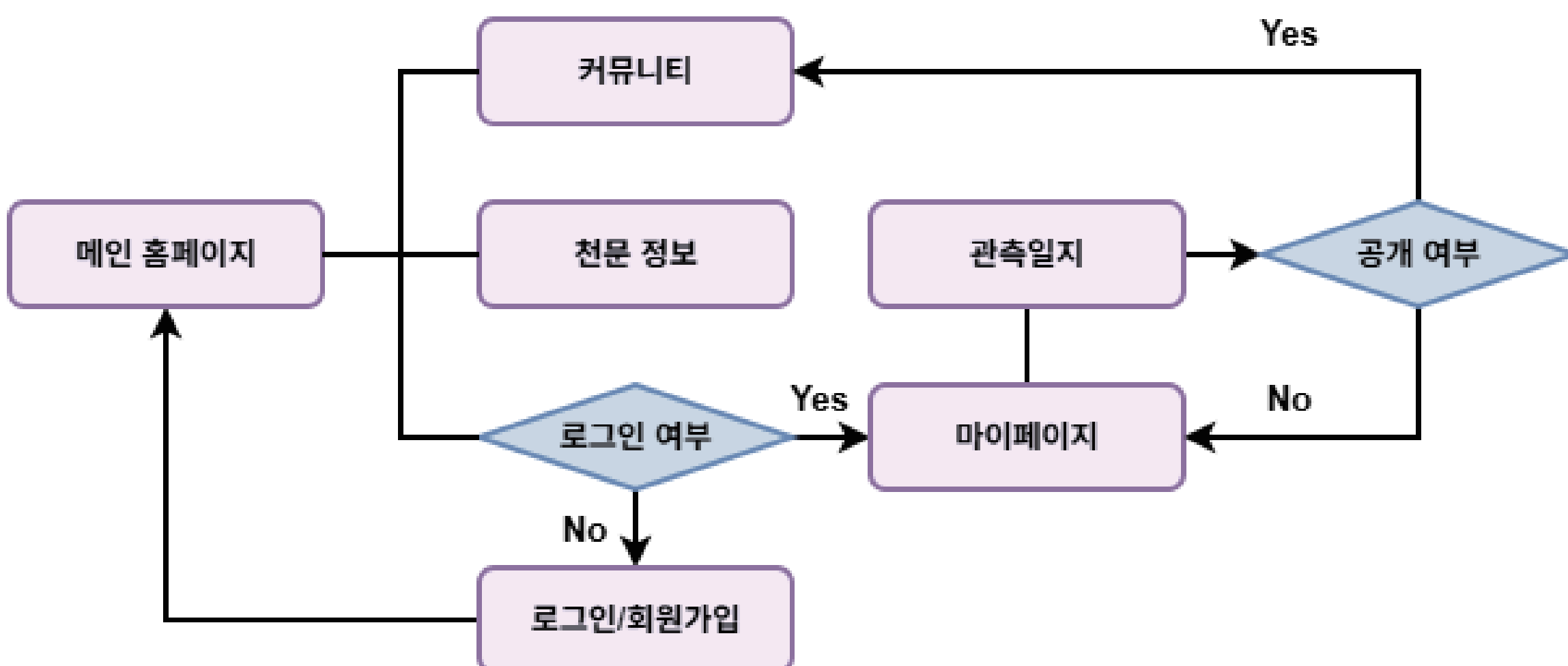
사용자 흐름도
