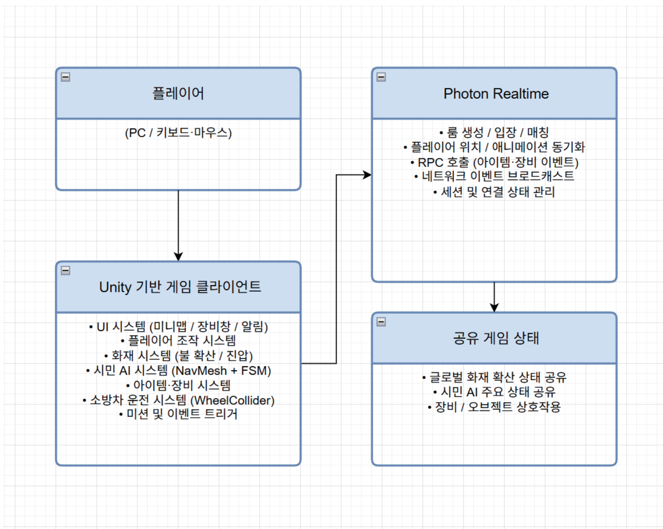
정보구조도
