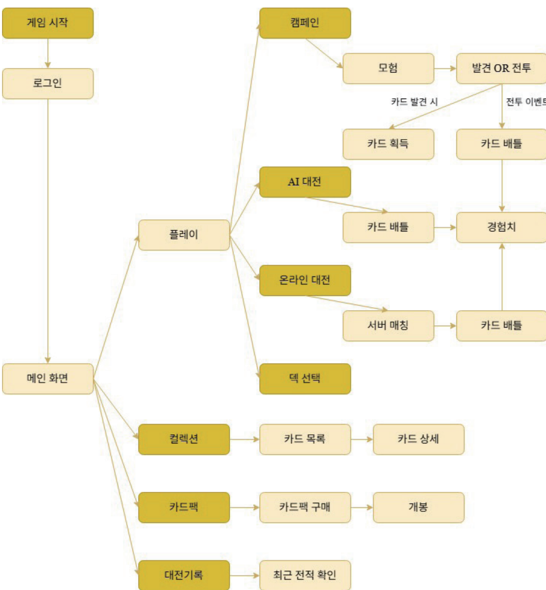
정보구조도
