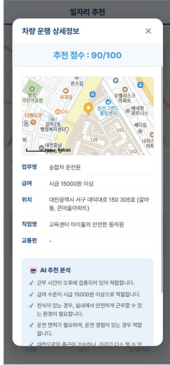
UI 이미지
