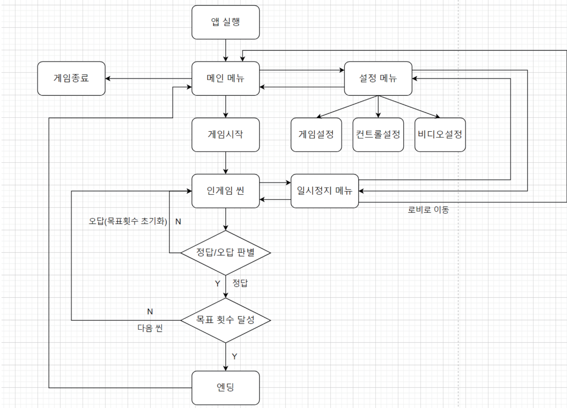
정보구조도
