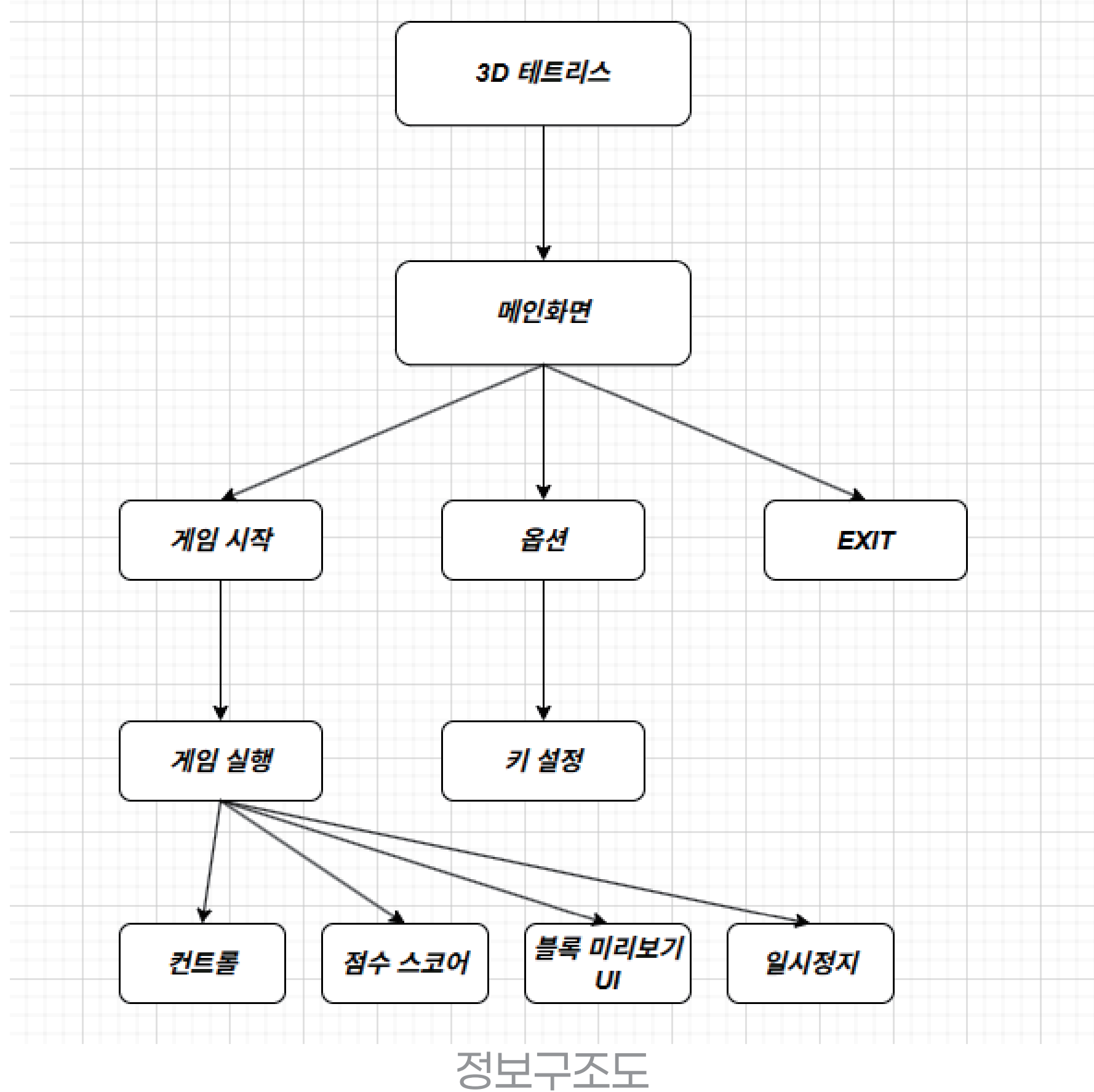
정보구조도
