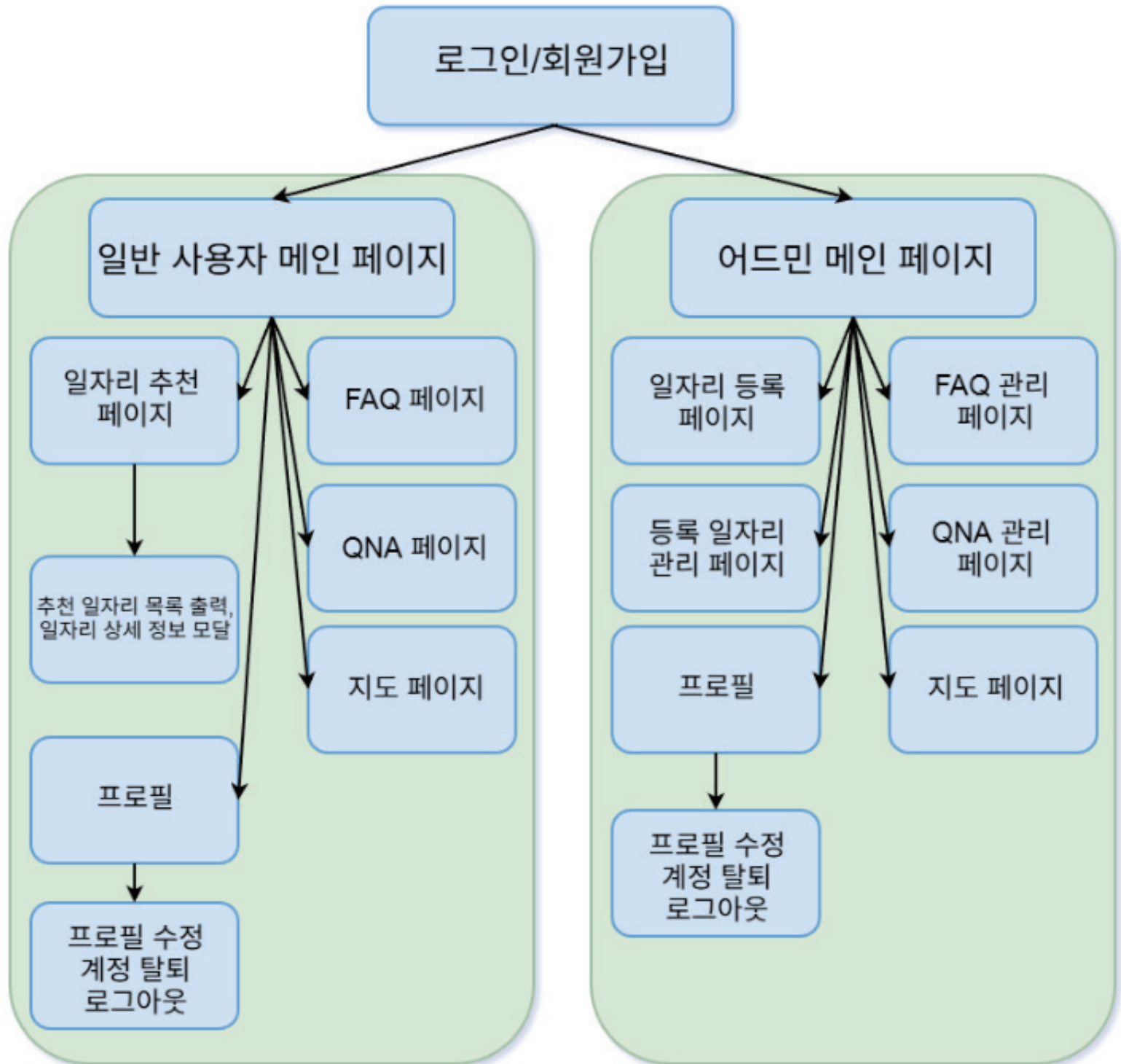
정보구조도
