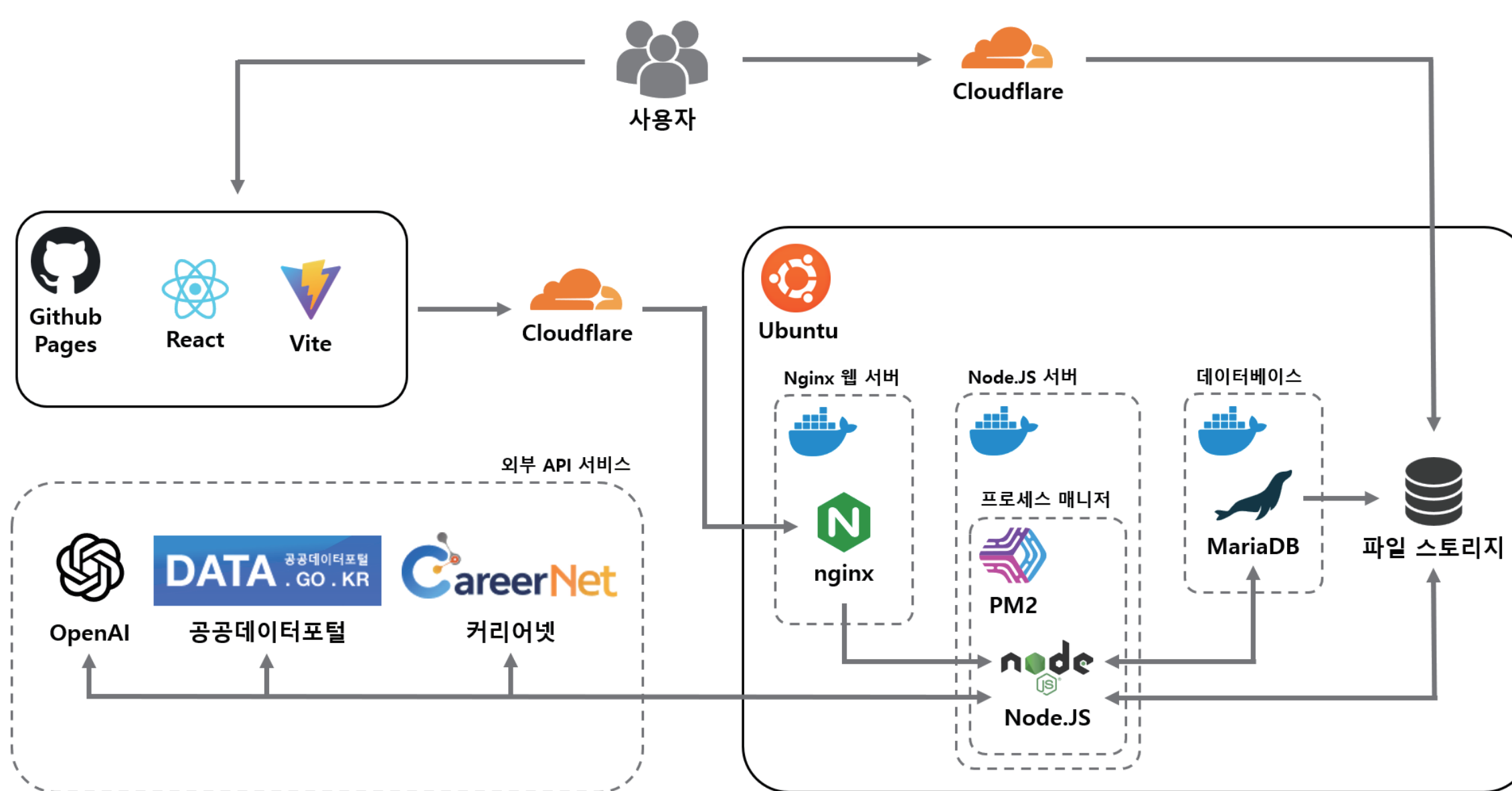
아키텍처 구조도
