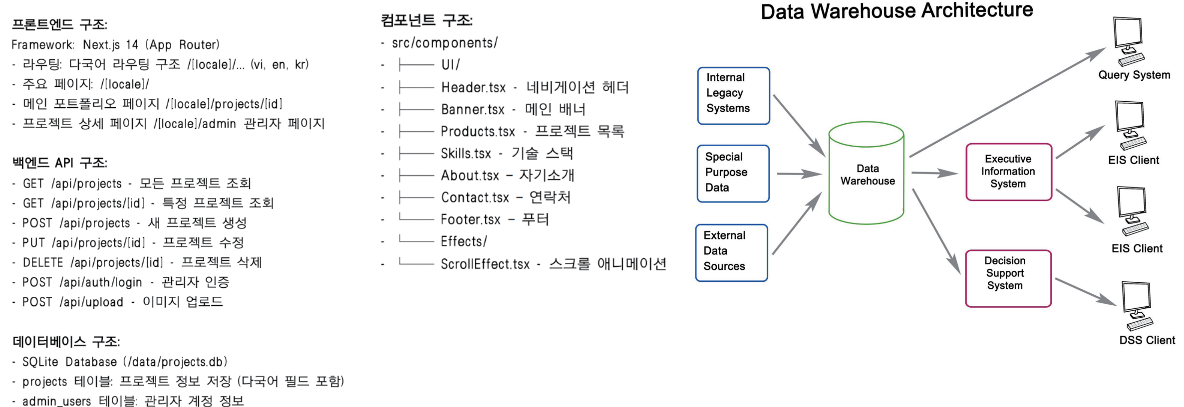
정보구조도
