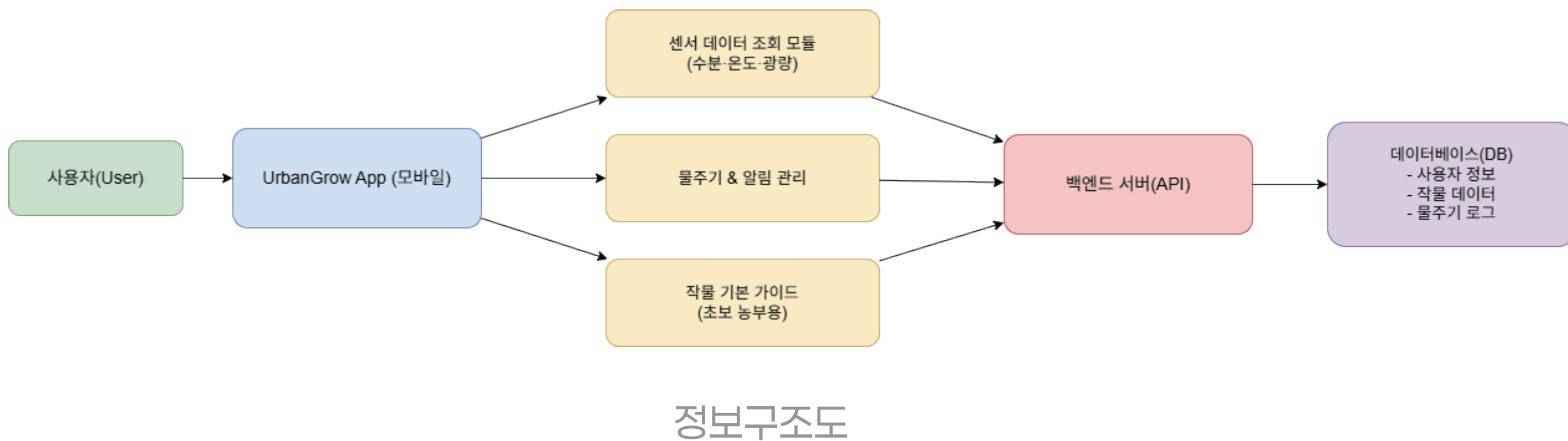
정보구조도
