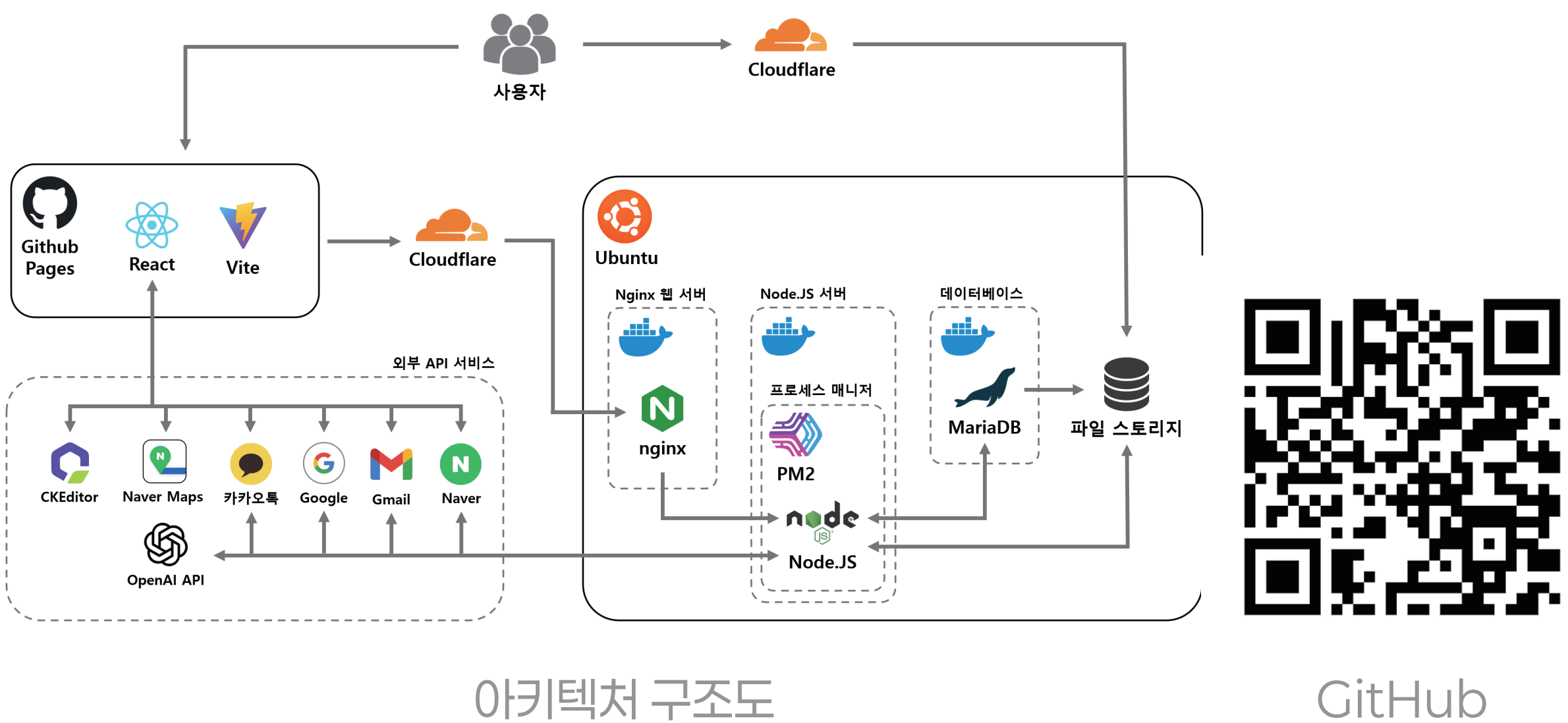
아키텍처 구조도
