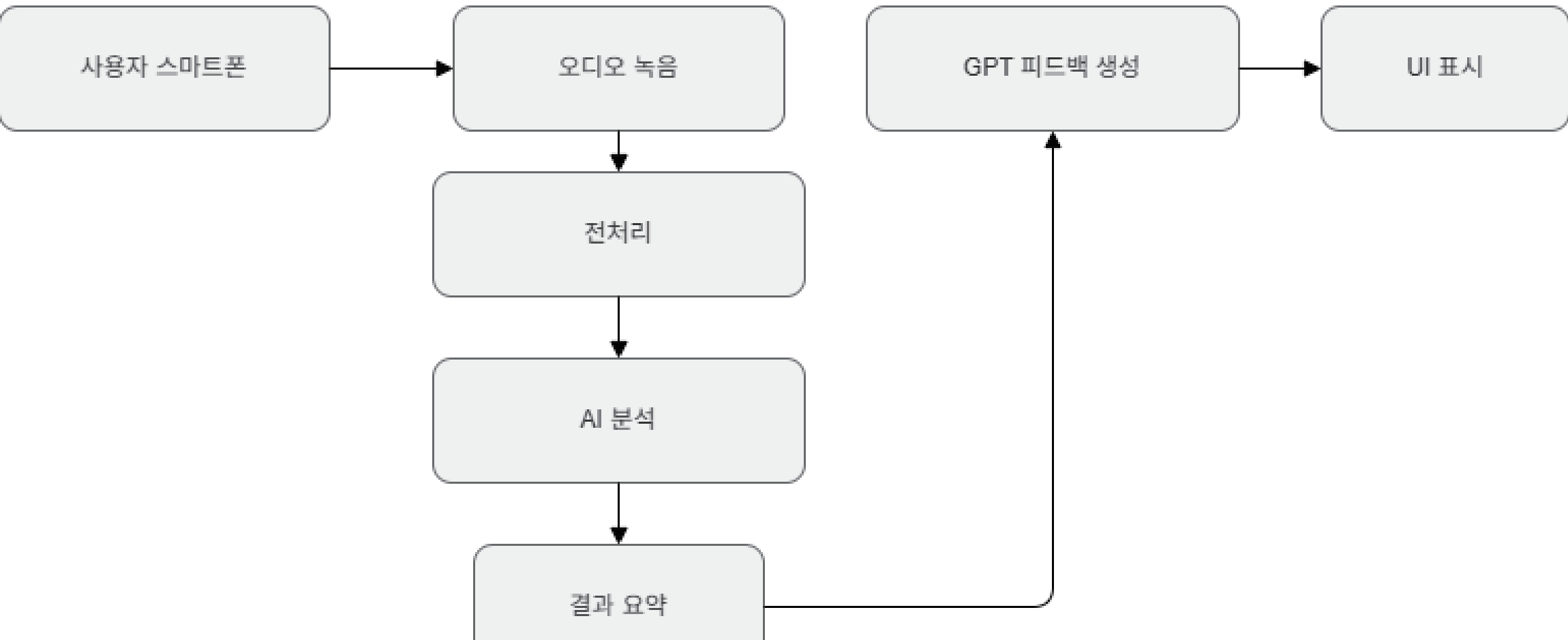
정보구조도
